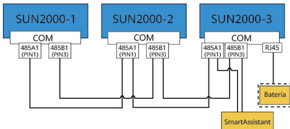
Figura 5-16 Conexión en red del SmartAssistant (los componentes opcionales están encerrados en recuadros de rayas pequeñas)
