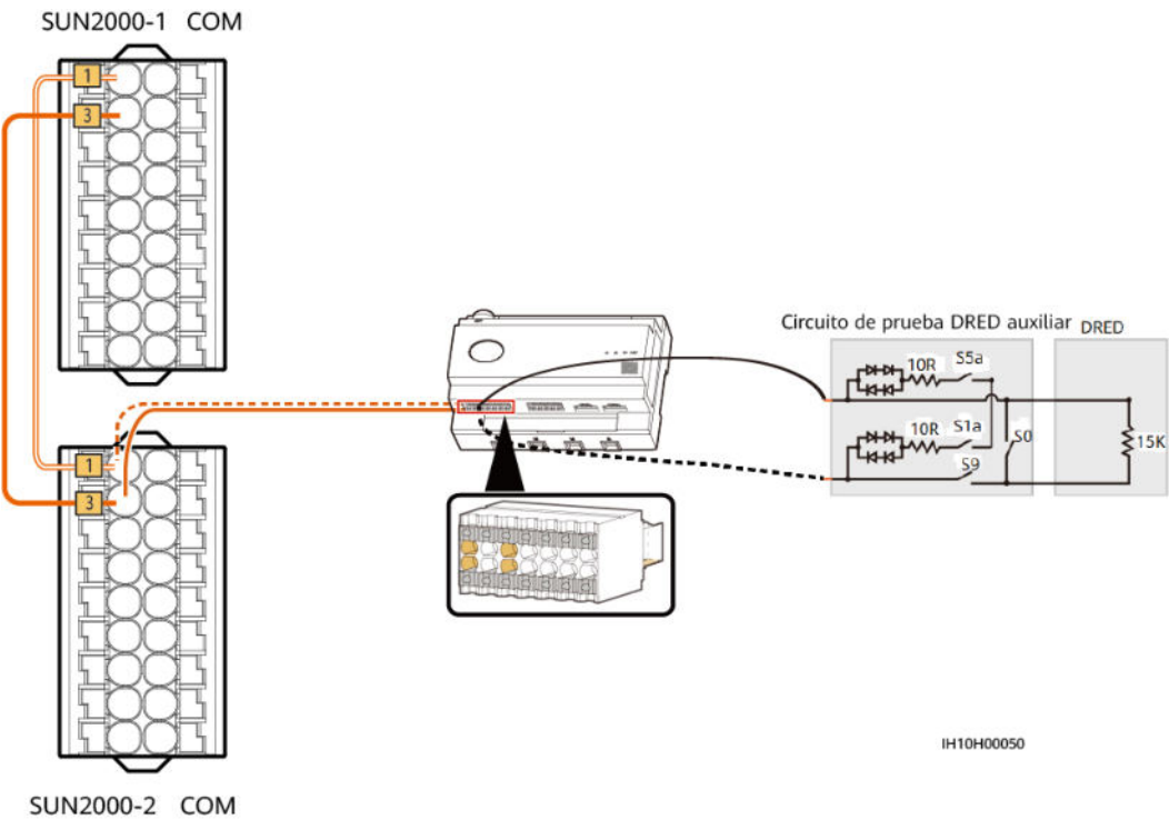
Figura 7-10 Diagrama de cableado para la función de DRM (conexión en red del SmartAssistant)
