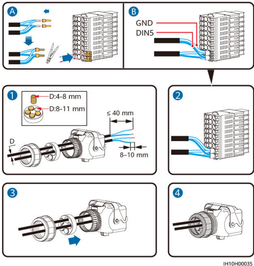
Figura 5-31 Instalación del cable
