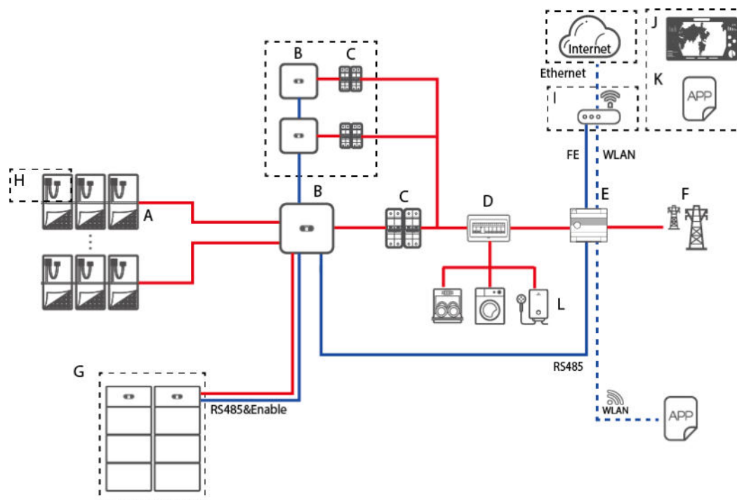
Figura 2-3 Conexión en red del SmartAssistant (los componentes opcionales están encerrados en recuadros de rayas pequeñas)
