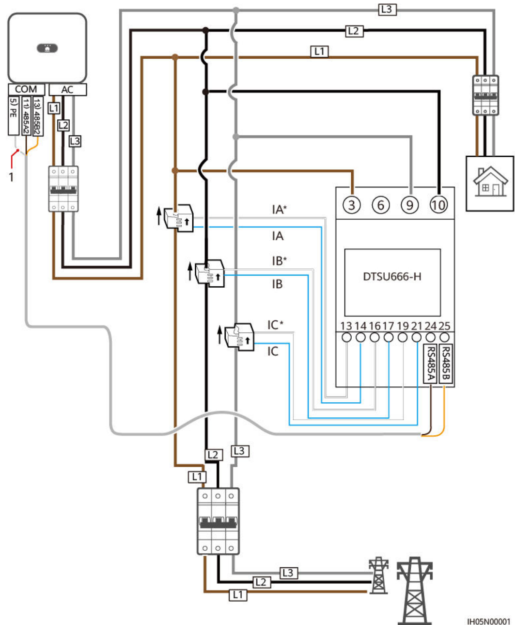
Figura 5-21 Conexión de cables trifásicos y trifilares del DTSU666-H (conexión en red del Smart Dongle)
