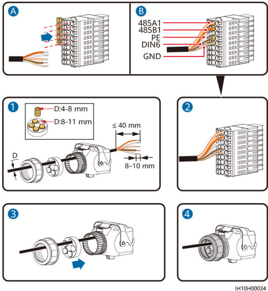
Figura 5-28 Instalación del cable
