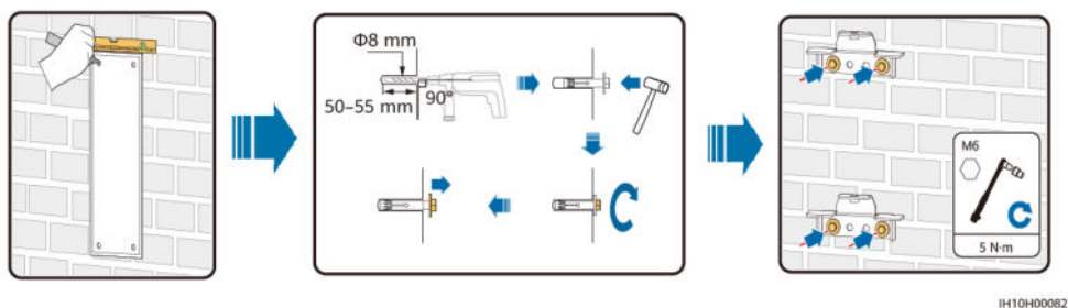
Figura 4-8 Instalación de las ménsulas de montaje
