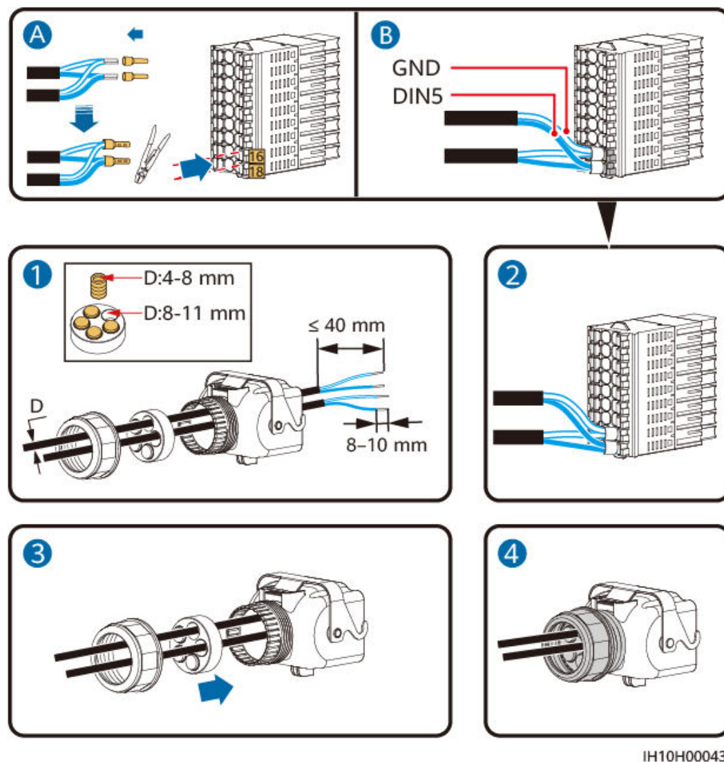
Figura 5-37 Instalación de los cables
