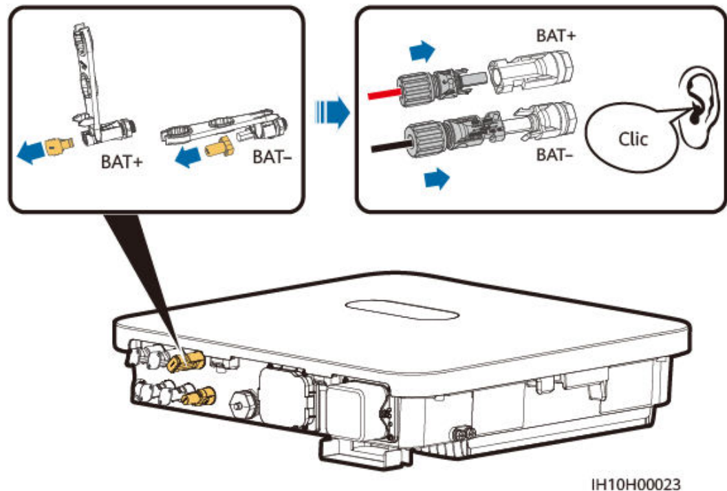
Figura 5-12 Conexión de los cables de la batería
