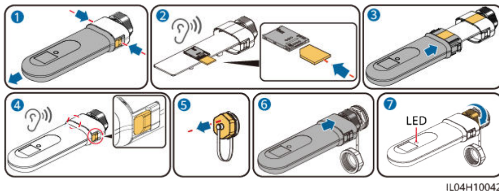
Figura 5-43 Instalación del Smart Dongle 4G (SDongleB-06)
