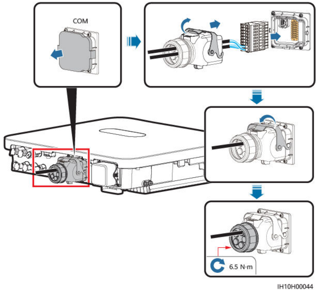
Figura 5-32 Fijación del conector del cable de señal
