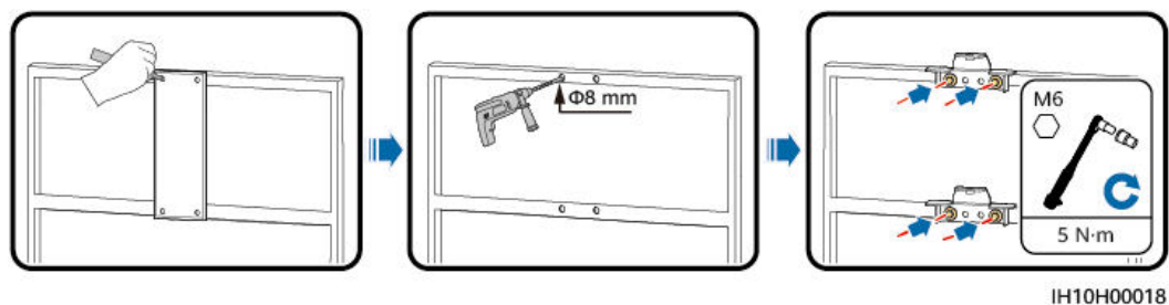
Figura 4-11 Instalación de las ménsulas de montaje
