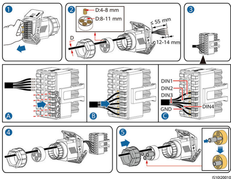
Figura 5-40 Instalación del cable
