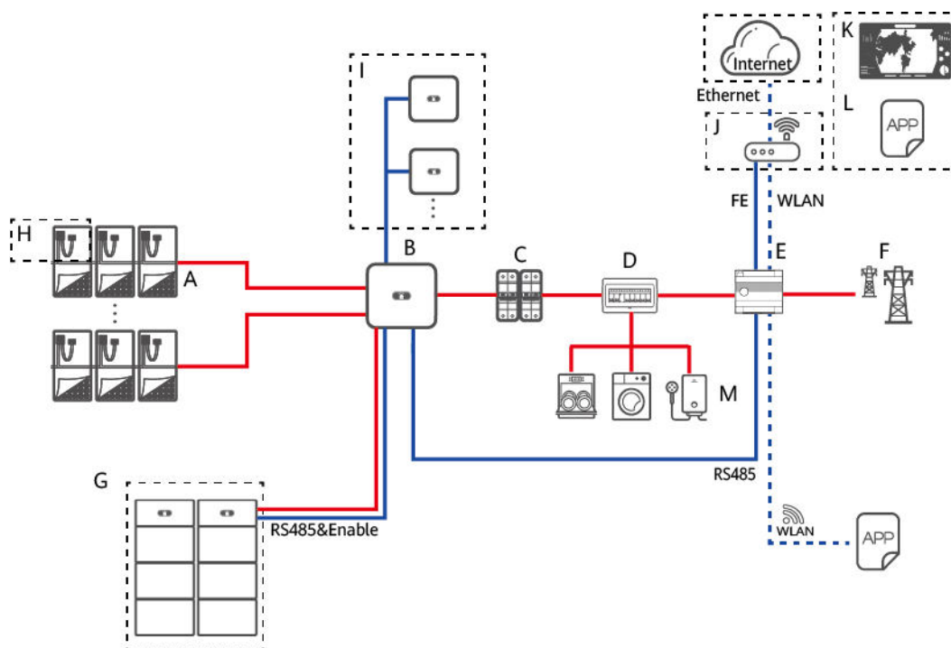
Figura 2-3 Conexión en red del SmartAssistant (los componentes opcionales están encerrados en cuadros de rayas pequeñas)
