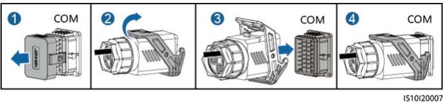
Figura 5-27 Cómo ajustar el conector del cable de señal
