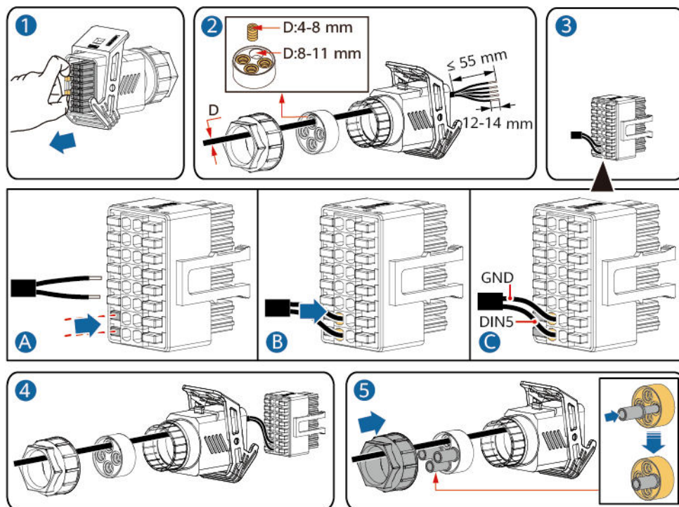
Figura 5-36 Cómo instalar el cable
