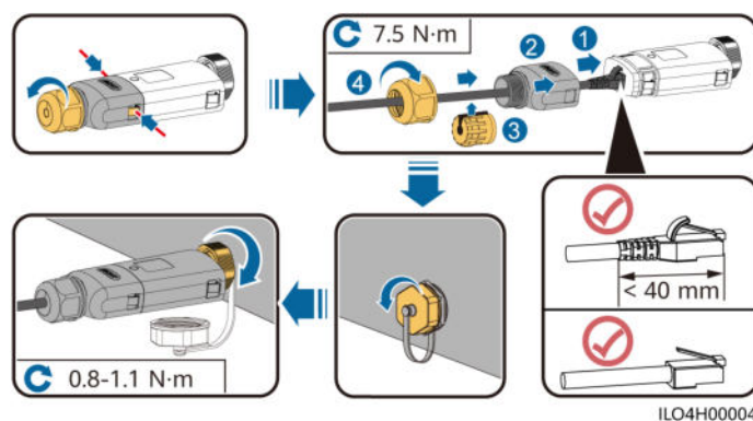
Figura 5-45 Instalación del Smart Dongle WLAN-FE (comunicación FE)
