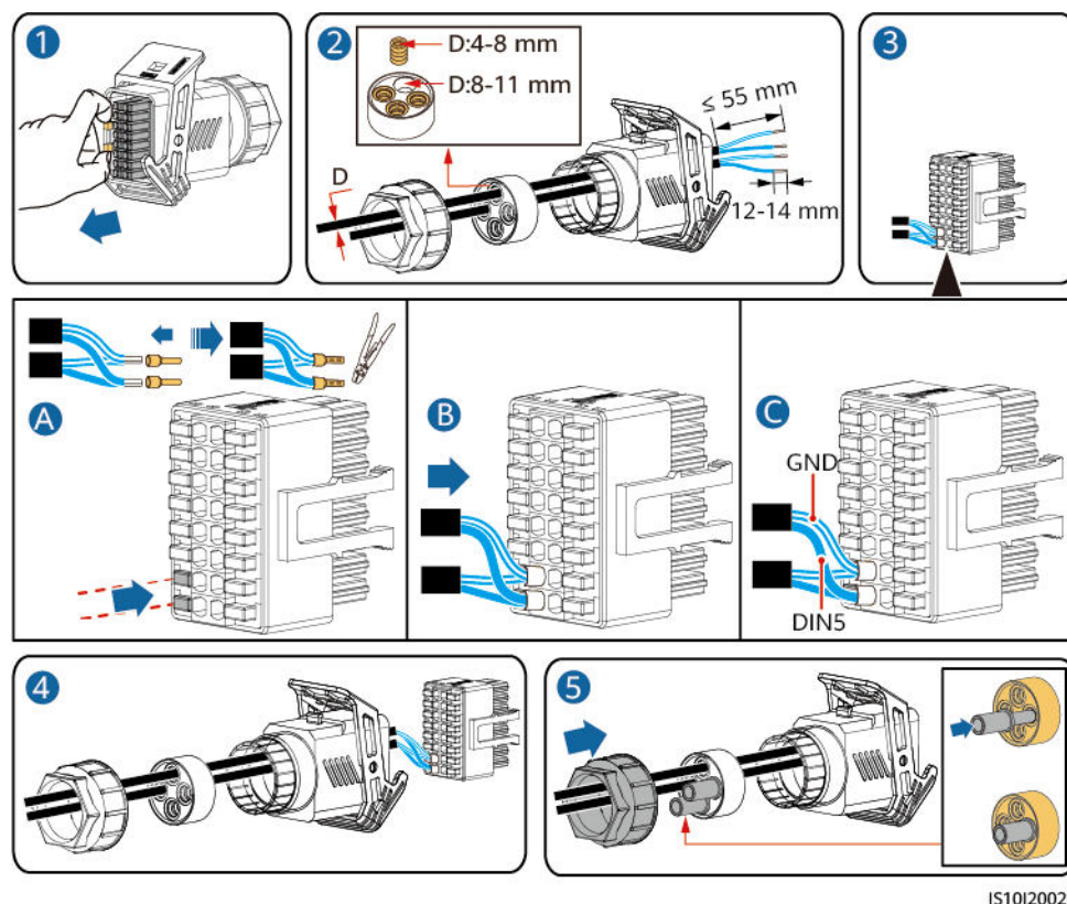
Figura 5-43 Instalación de los cables
