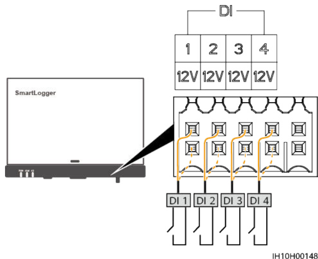
Figura 5-39 Conexiones de los cables (conexión a red del SmartLogger)
