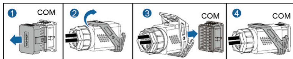
Figura 5-29 Fijación del conector del cable de señal
