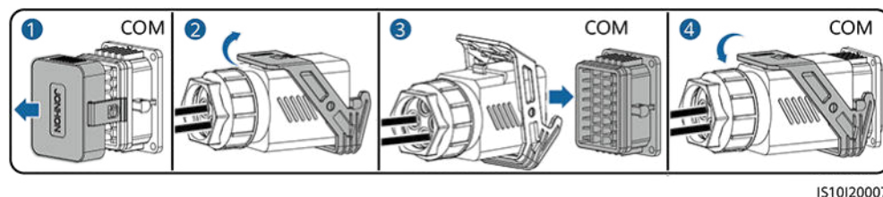
Figura 5-44 Fijación del conector del cable de señal
