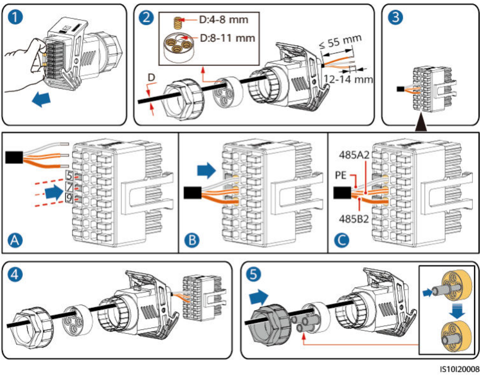
Figura 5-26 Cómo instalar el cable
