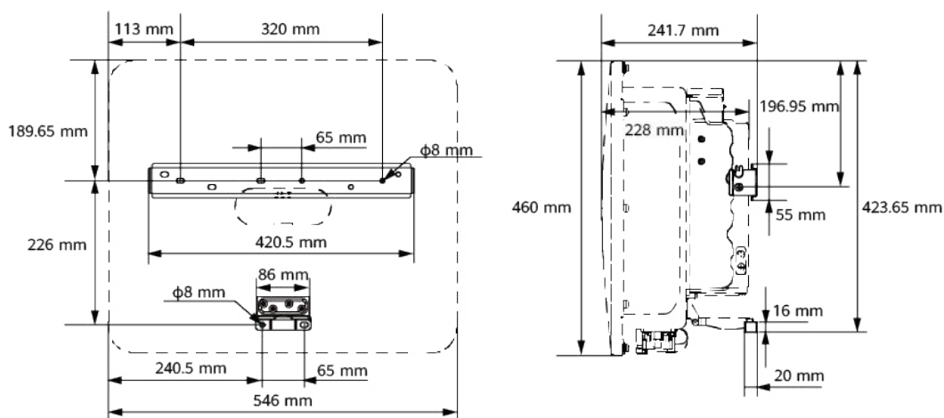
Figura 4-1 Dimensiones del inversor y de la ménsula de montaje
