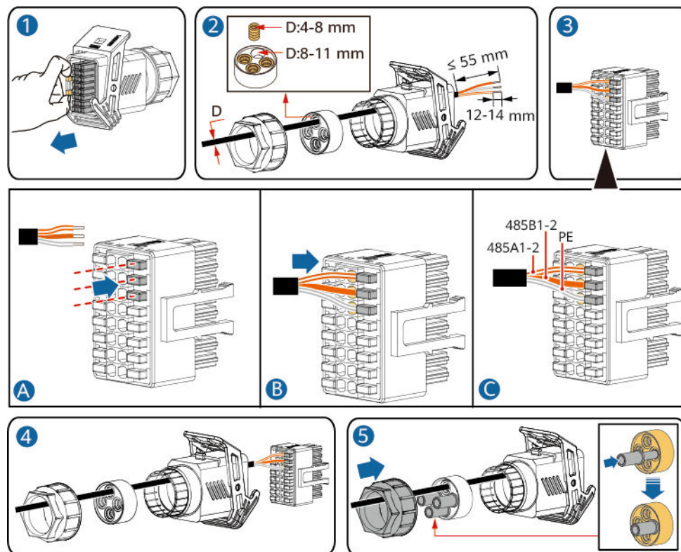
Figura 5-30 Instalación del cable
