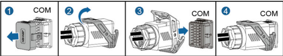
Figura 5-33 Fijación del conector del cable de señal
