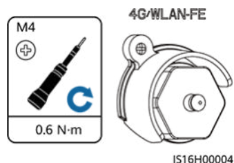
Figura 5-48 Instalación de componentes antirrobo para el Smart Dongle
