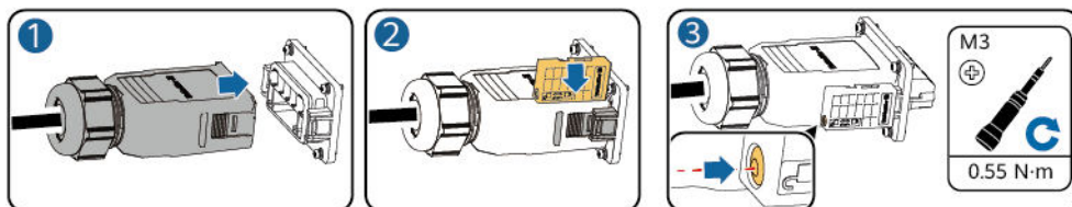
Figura 5-9 Fijación del conector de CA
