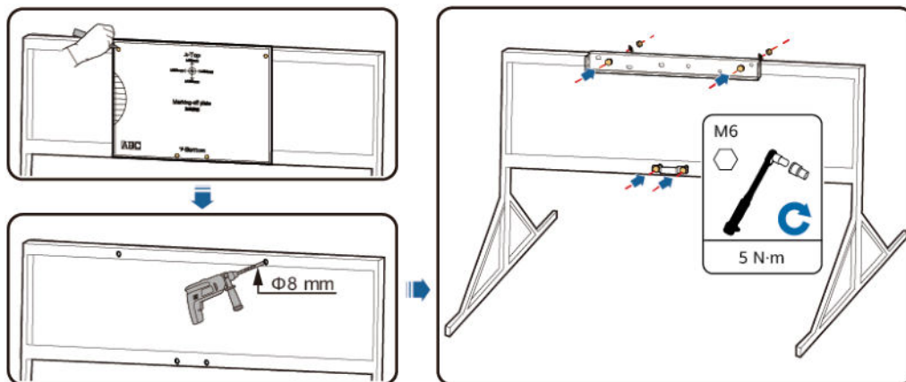
Figura 4-9 Fijación de la ménsula de montaje
