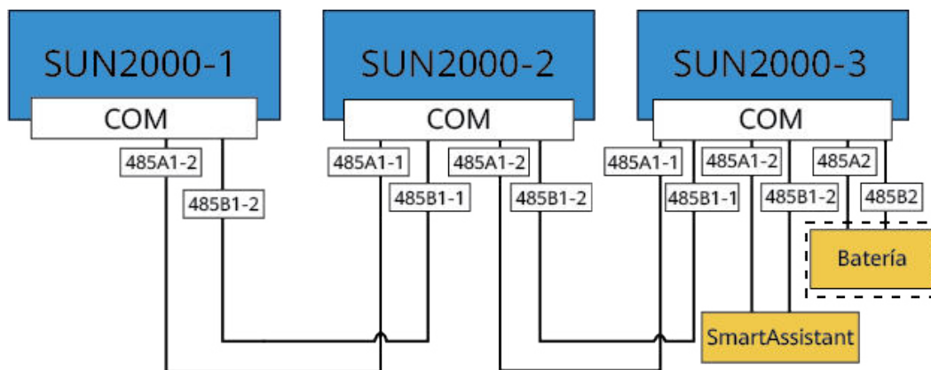
Figura 5-19 Conexión en red del SmartAssistant (los componentes opcionales están encerrados en cuadros de rayas pequeñas)
