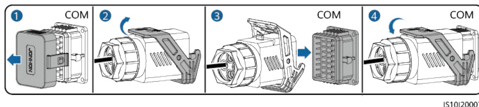
Figura 5-41 Fijación del conector del cable de señal
