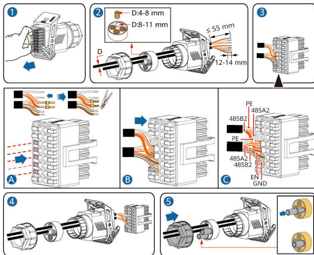
Figura 5-28 Instalación de los cables
