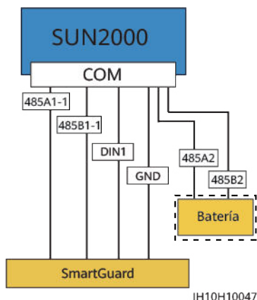
Figura 5-20 Conexión en red del SmartGuard (los componentes opcionales están encerrados en cuadros de rayas pequeñas)
