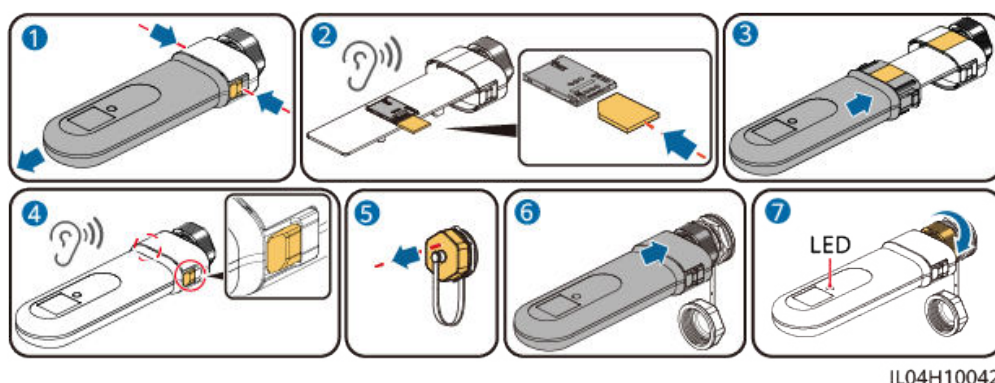
Figura 5-47 Instalación del Smart Dongle 4G (SDongleB-06)
