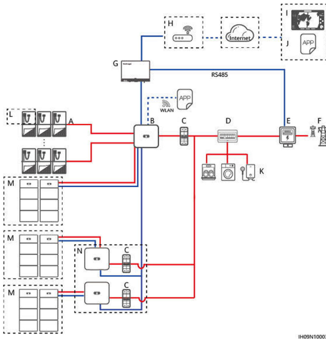
Figura 2-6 Conexión en red del SmartLogger (los componentes opcionales están encerrados en cuadros de rayas pequeñas)
