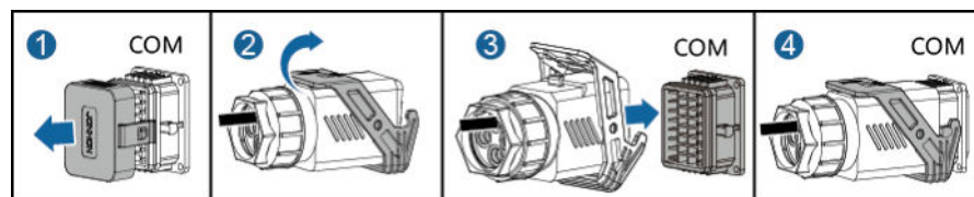
Figura 5-31 Fijación del conector del cable de señal
