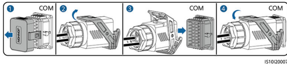
Figura 5-22 Cómo ajustar el conector del cable de señal
