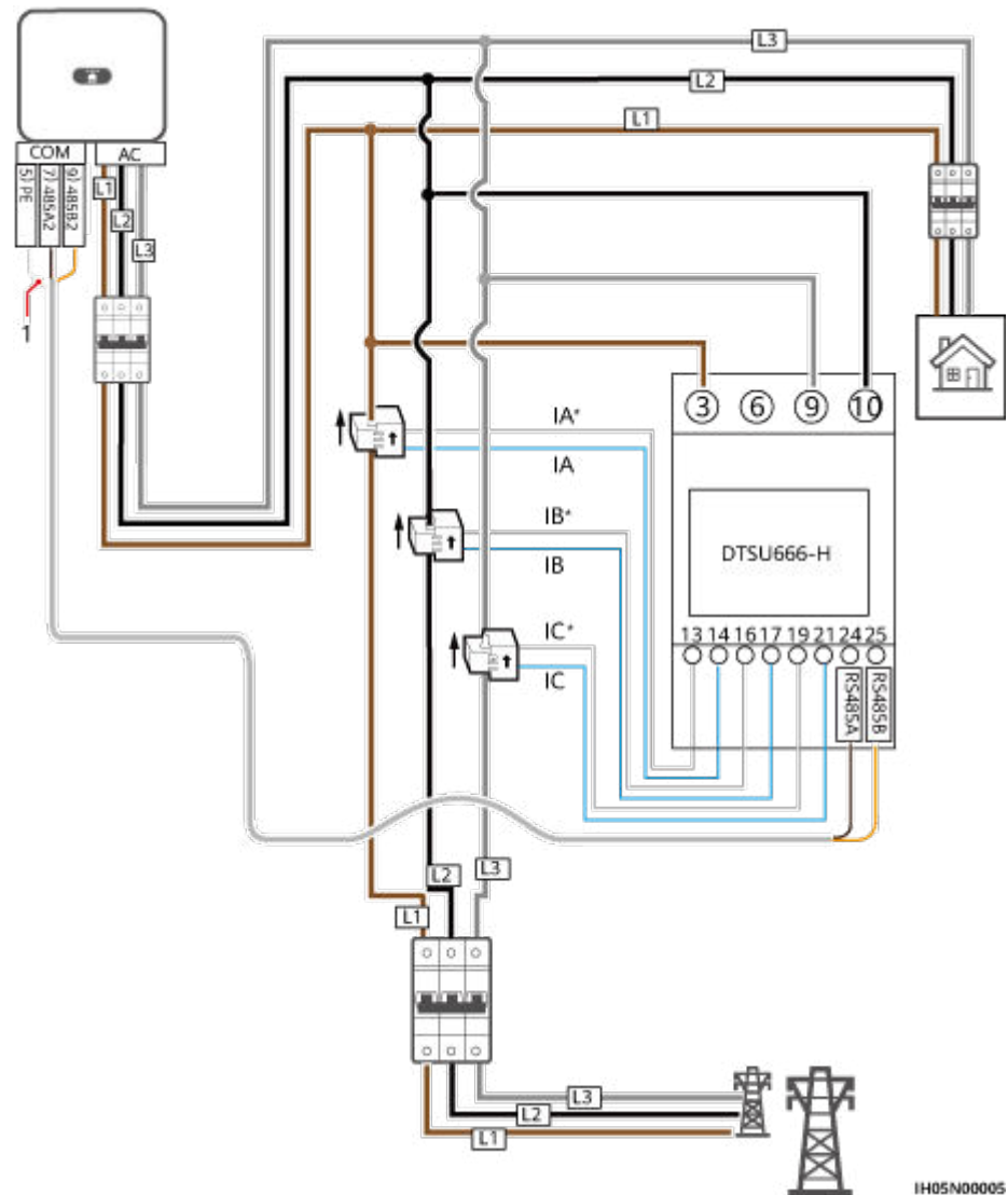
Figura 5-23 Conexión de cables trifásicos y trifilares del DTSU666-H (conexión en red del Smart Dongle)
