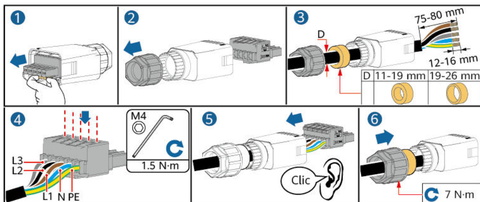
Figura 5-8 Cable de cinco conductores (L1, L2, L3, N y PE)
