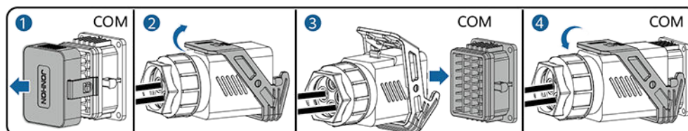
Figura 5-33 Fijación del conector del cable de señal
