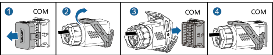
Figura 5-36 Cómo ajustar el conector del cable de señal
