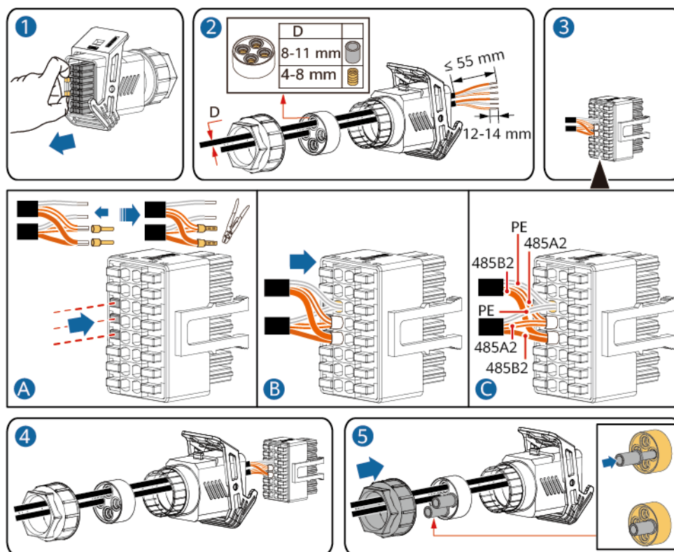
Figura 5-32 Instalación del cable
