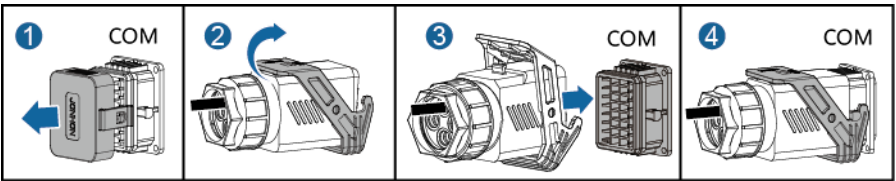
Figura 5-38 Fijación del conector del cable de señal
