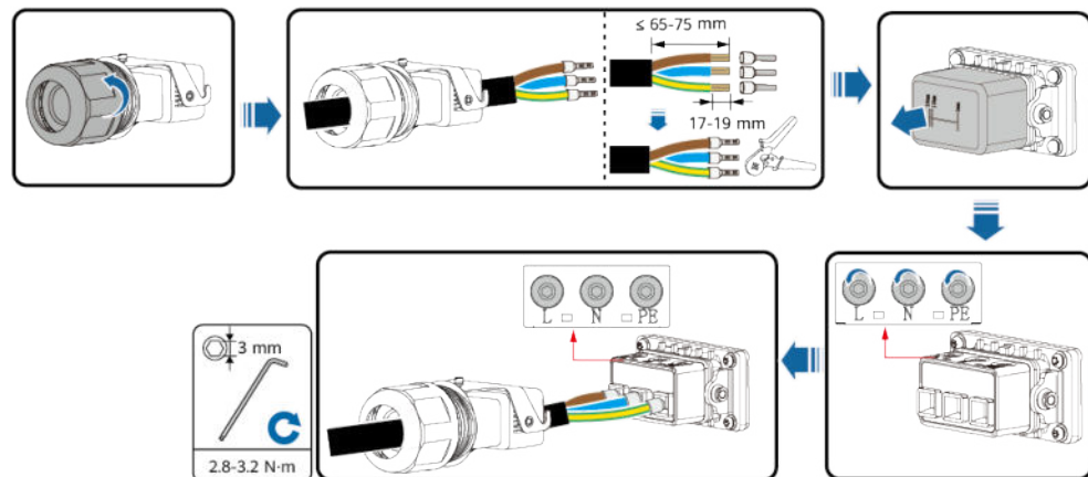
Figura 5-4 Instalación del cable de alimentación de CA
