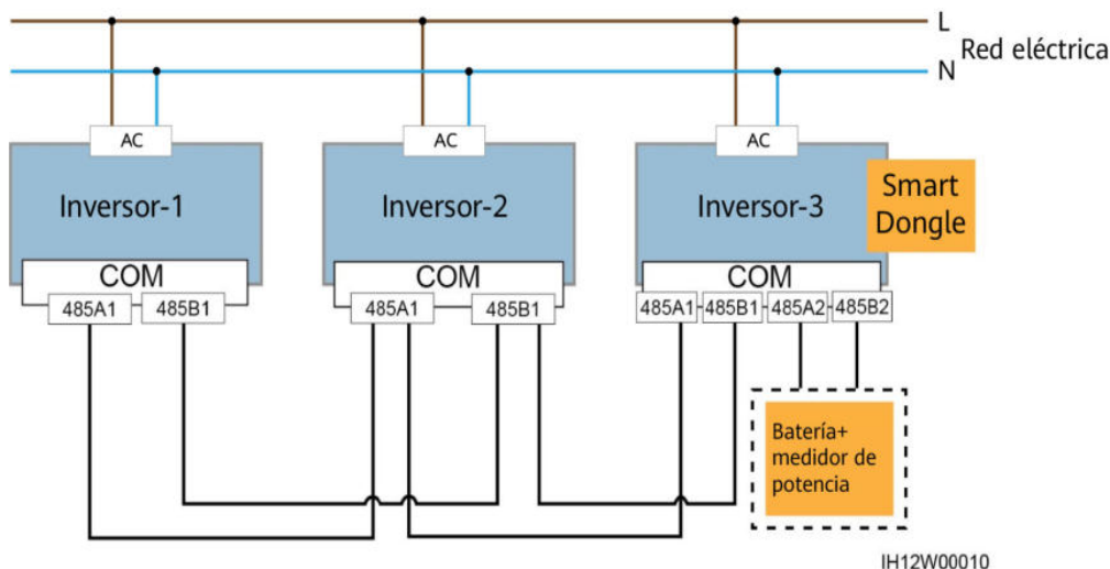
Figura 5-14 Conexión en red del Smart Dongle (los componentes opcionales están encerrados en el cuadro de rayas pequeñas)
