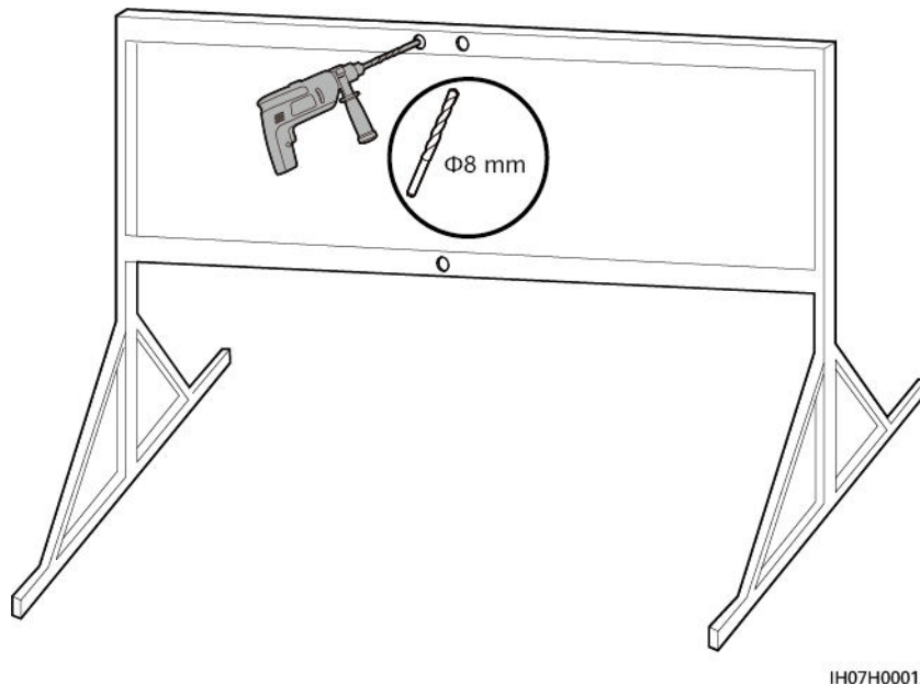
Figura 4-12 Perforación de orificios
