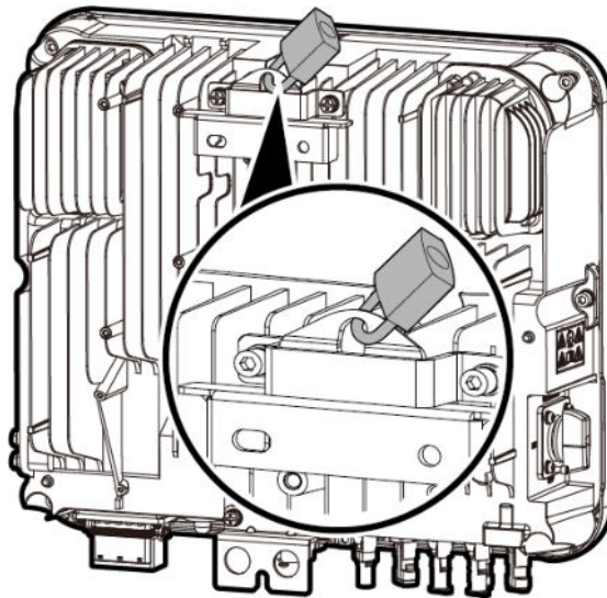
Figura 4-10 Instalación de un candado antirrobo
