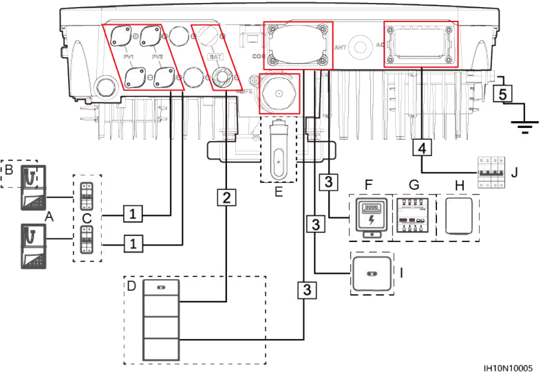
Figura 5-1 Conexiones de los cables del inversor (los componentes encerrados en recuadros de rayas pequeñas son opcionales)
