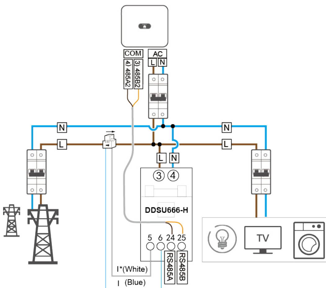
Figura 5-28 Conexión de los cables al medidor de potencia DDSU666-H
