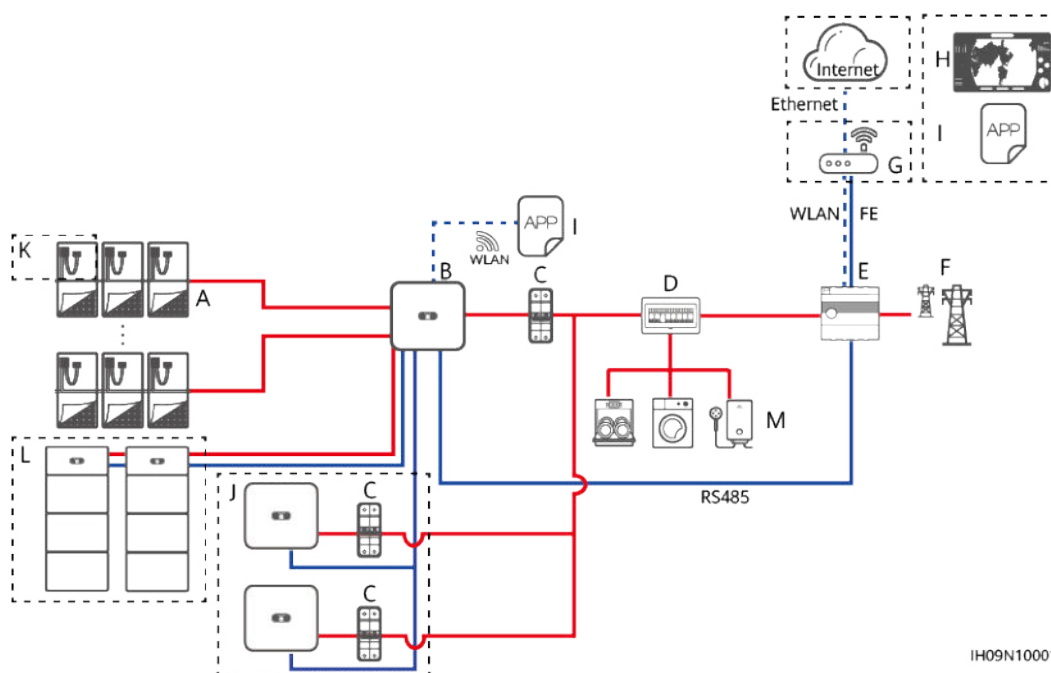
Figura 2-2 Conexión en red del SmartAssistant (los componentes opcionales están encerrados en recuadros de rayas pequeñas)
